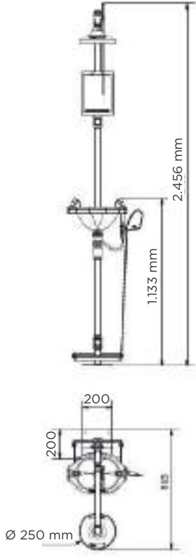
DATOS TÉCNICOS 12027
