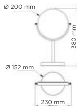
DATOS TÉCNICOS 05142
