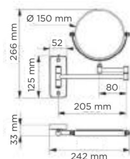
DATOS TÉCNICOS 05023
