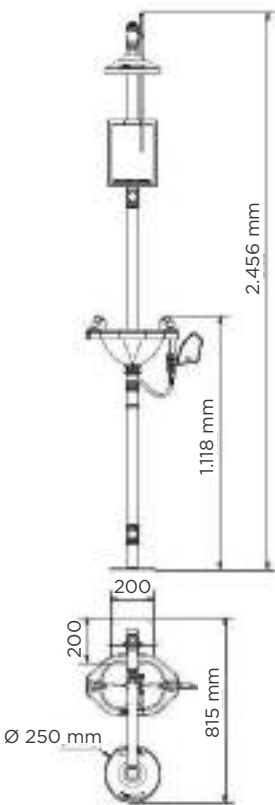
DATOS TÉCNICOS 12025
