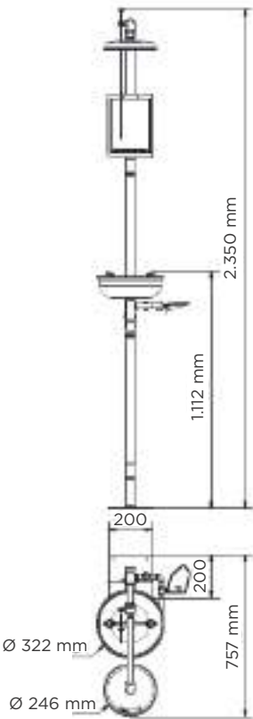
DATOS TÉCNICOS 12026
