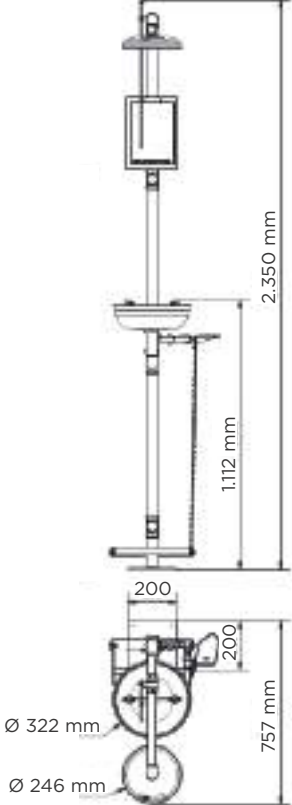
DATOS TÉCNICOS 12028
