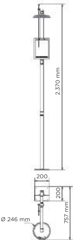
DATOS TÉCNICOS 12024
